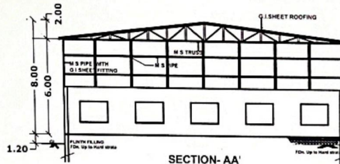
SECTION-AA' (SCALE-1:200)
